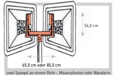
zwei Spiegel an einem Rohr-, Mauerpfosten oder Wandarm
