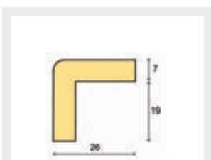
Kantenschutz Winkel, Typ E
