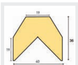
Kantenschutz Trapez, Typ AA
