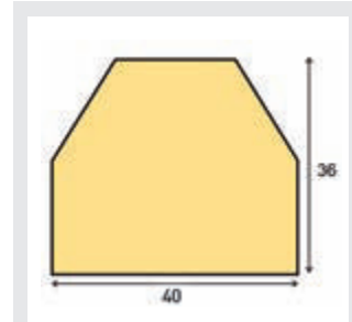
Flächenschutz Trapez, Typ CC
